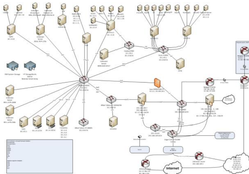
Схема центрального ЦОДа МГППУ
