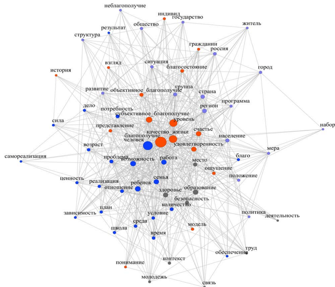
Смысловые ассоциации вокруг понятия "благополучие". Цветом обозначены смысловые кластеры на основе построенной семантической сети. Размер точки — оценка семантической близости к категории "благополучие", выраженному в количестве сильных связей (метрика closeness centrality)
